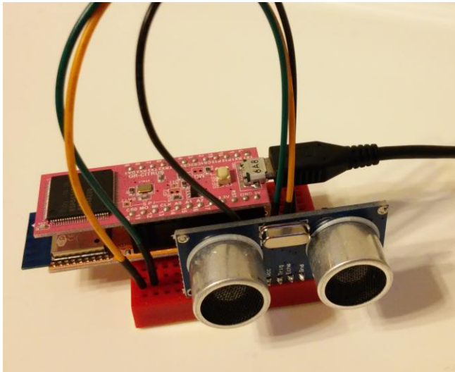
GR-CITRUS+WA-MIKAN 超音波センサー
